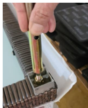
Gewindestange im Tischrahmen festziehen
